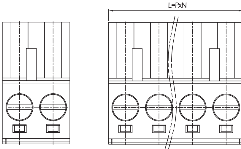
2 Pole Module
